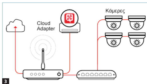
3 Η αρχιτεκτονική του ADESCO Video με σύνδεση μέσω IP καμερών.
