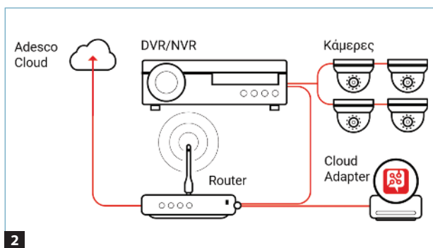
2 Η αρχιτεκτονική του ADESCO Video με σύνδεση μέσω DVR/NVR.
